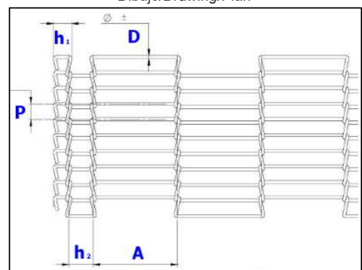
Dibujo/Drawing/Plan
